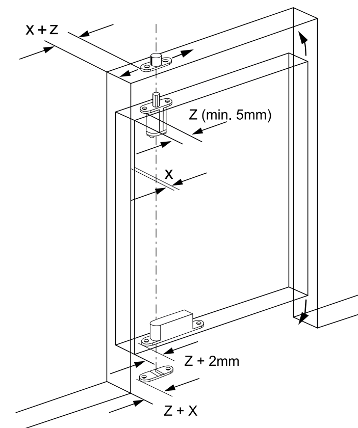
Завіси Pivotica дозволяють монтувати двері без коробки. При цьому вісь обертання можна зміщувати.
